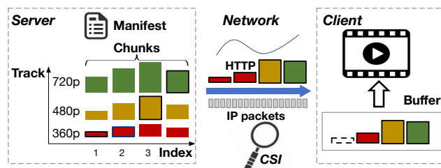
Figure 1. ABR streaming overview
