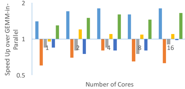
(d) Speed up of Stencil-Kernel (FP) over GEMM-in-Parallel.
